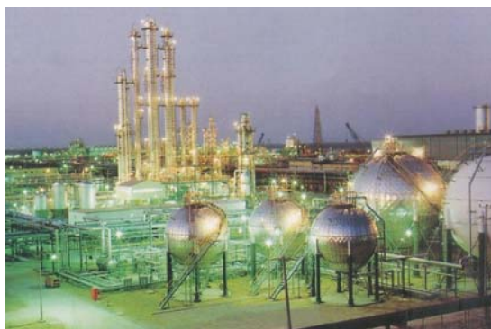
شکل ۱۷-۵ تاسیسات پتروشیمی بندر امام خمینی
